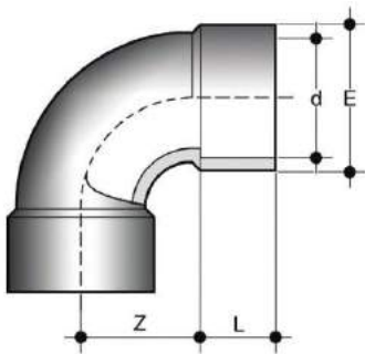
GIV Отвод 90°
